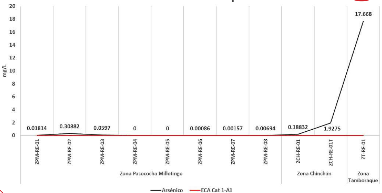
Gráfico N° 19. Valores de arsénico según Prueba de Lixiviados de Corto Plazo.
