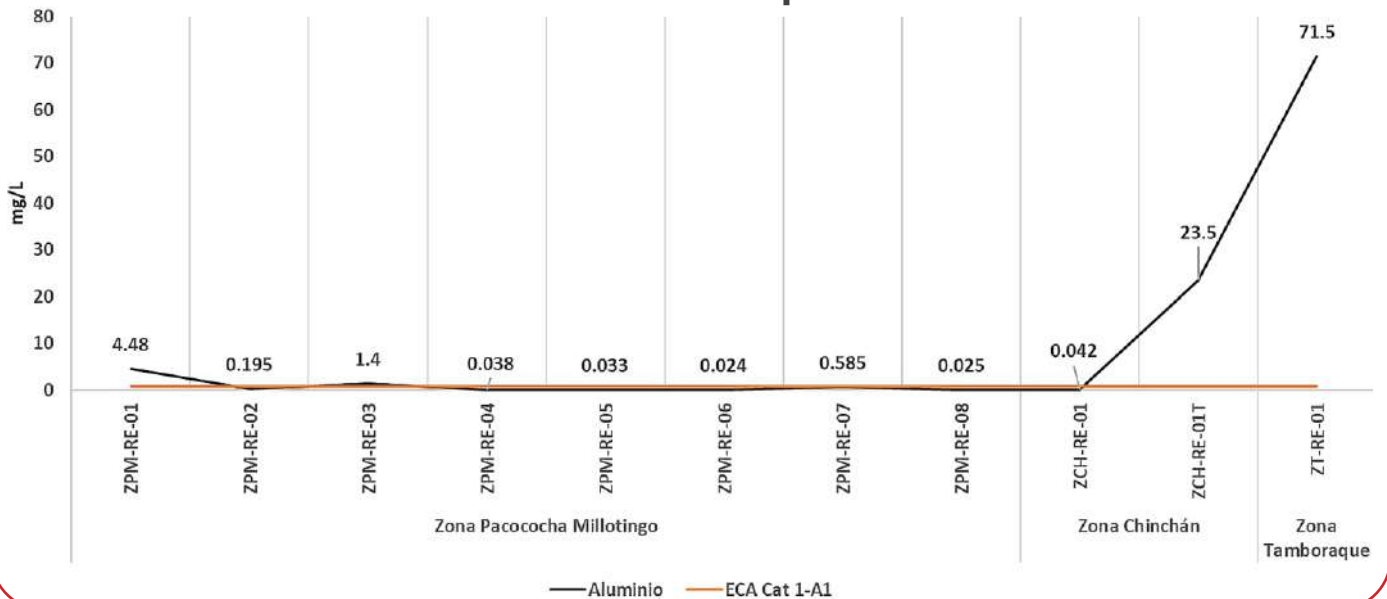
Gráfico N° 17. Valores de aluminio según Prueba de Lixiviados de Corto Plazo.
