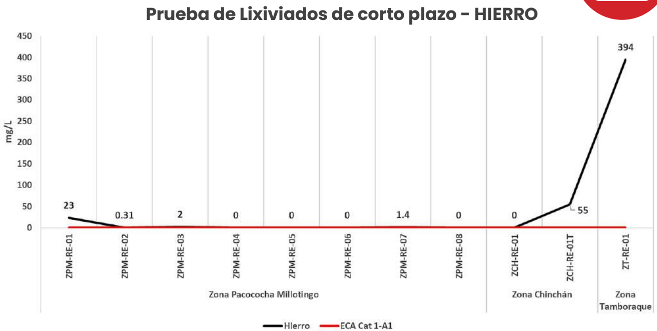
Gráfico N° 23. Valores de hierro según Prueba de Lixiviados de Corto Plazo
