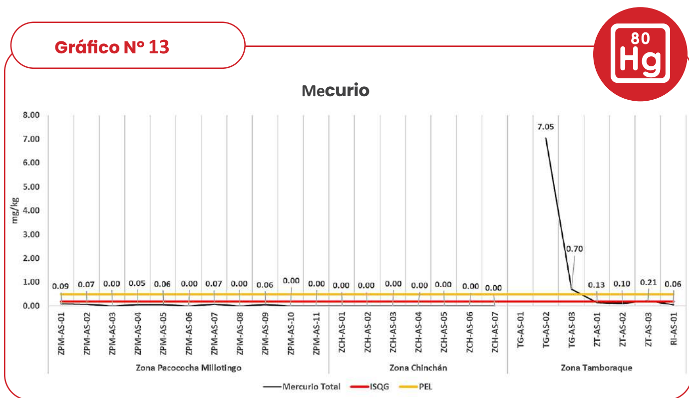
Gráfico N° 13. Valores de mercurio en sedimentos para las tres zonas.
