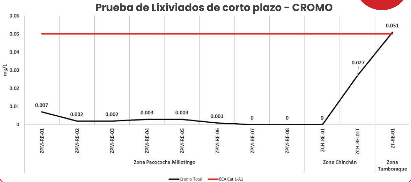
Gráfico N° 22. Valores de cromo según Prueba de Lixiviados de Corto Plazo.
