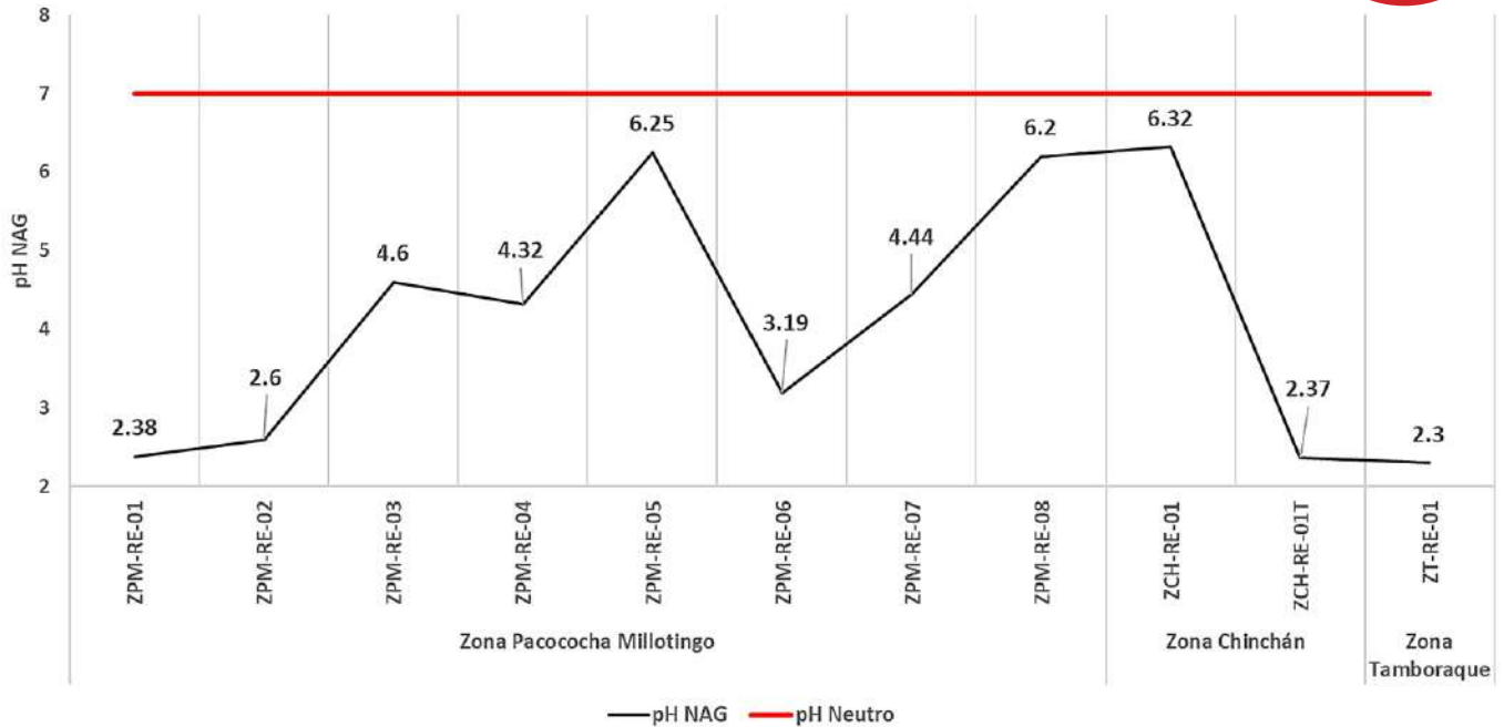
Gráfico N° 16. Valores de pH según el Potencial de Generación de Acidez (NAG).
