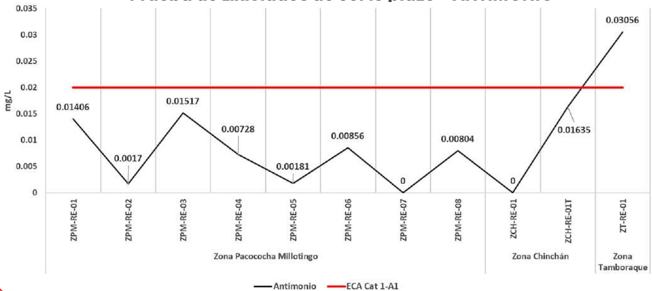
Gráfico N° 18. Valores de antimonio según Prueba de Lixiviados de Corto Plazo.
