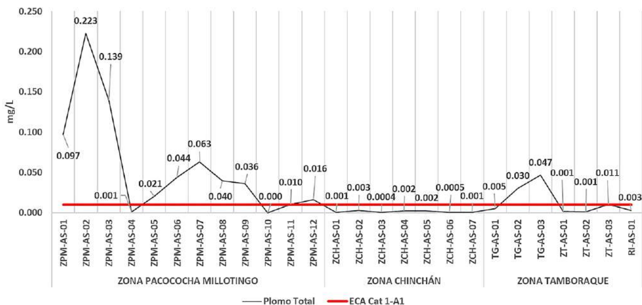
Gráfico N° 08. Valores de plomo en aguas superficiales para las tres zonas.
