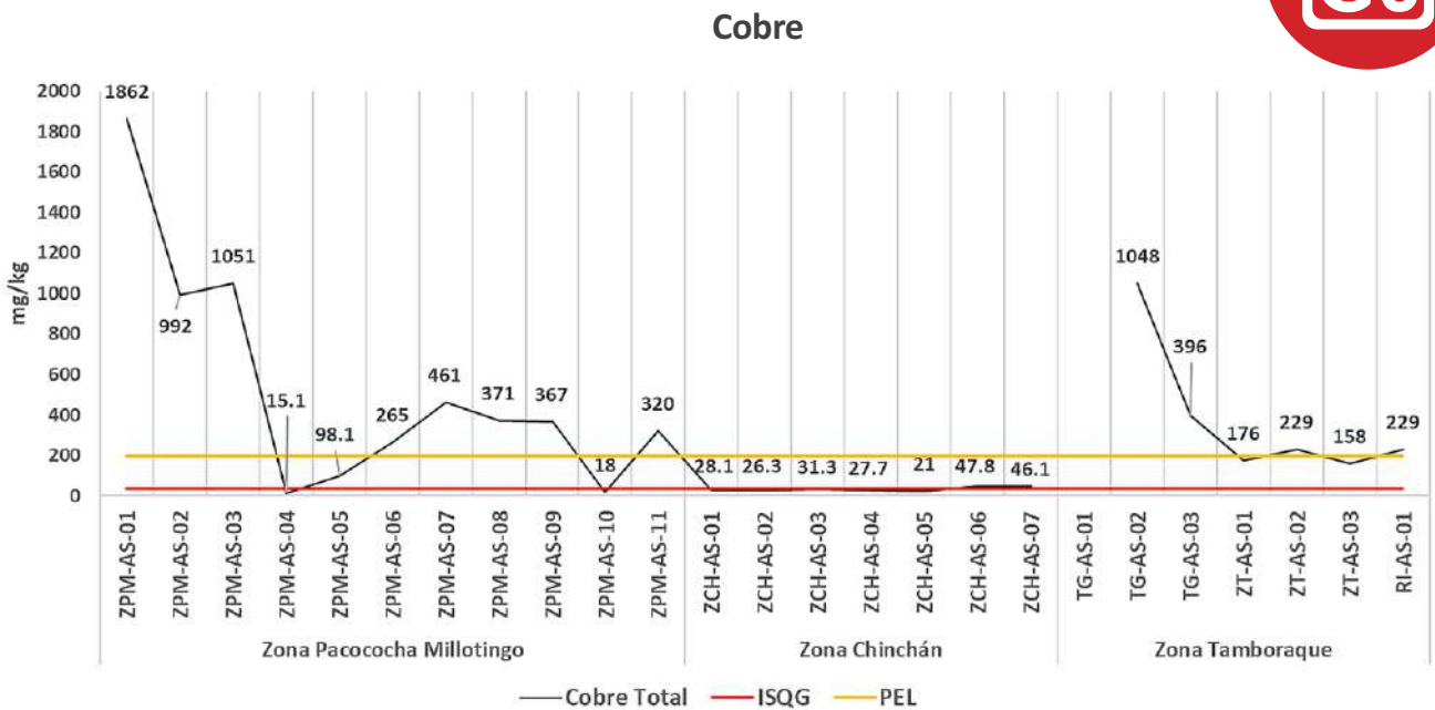
Gráfico N° 12. Valores de cobre en sedimentos para las tres zonas.
