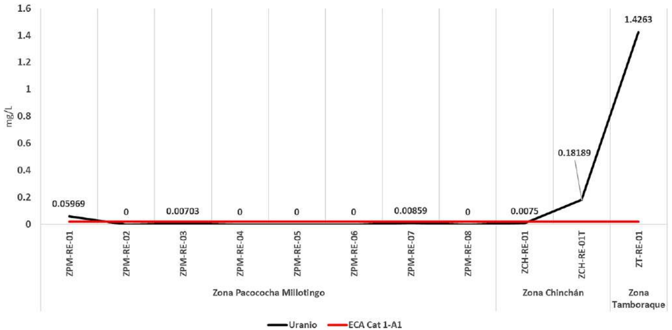
Gráfico N° 27. Valores de uranio según Prueba de Lixiviados de Corto Plazo
