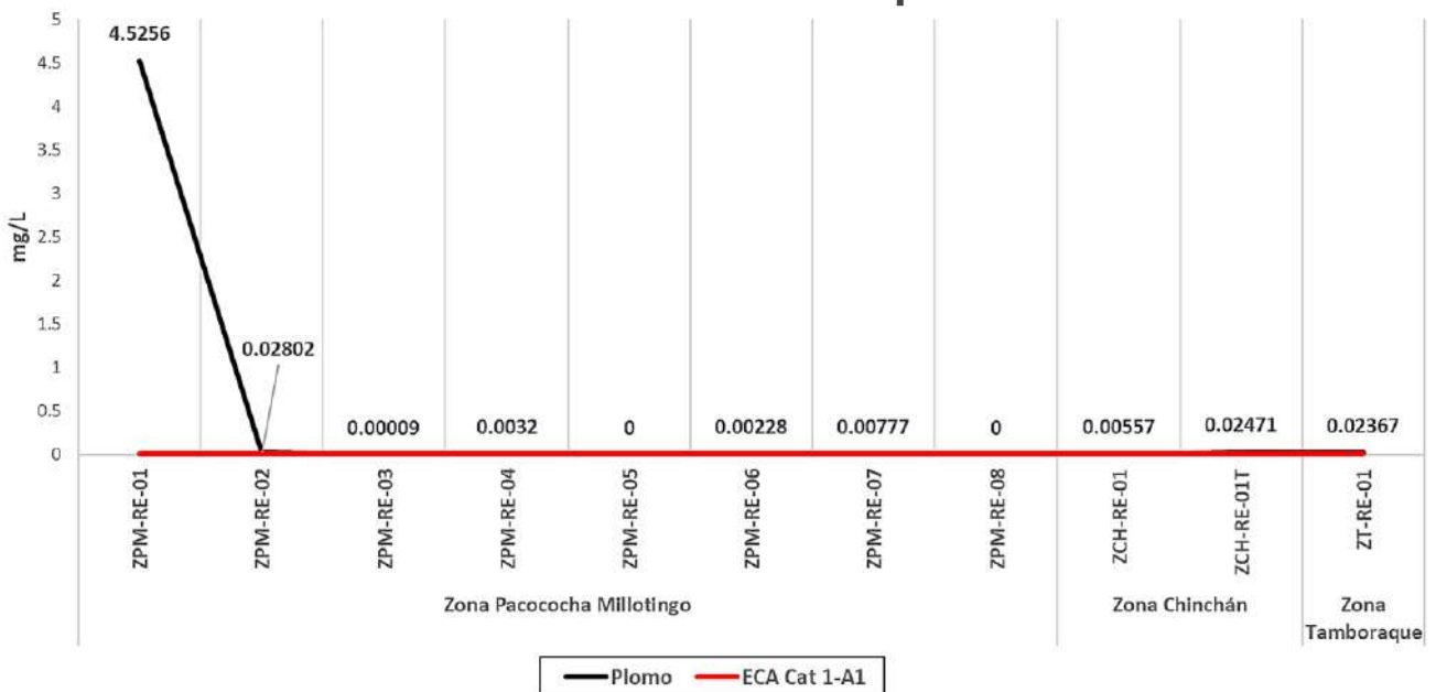
Gráfico N° 26. Valores de plomo según Prueba de Lixiviados de Corto Plazo.
