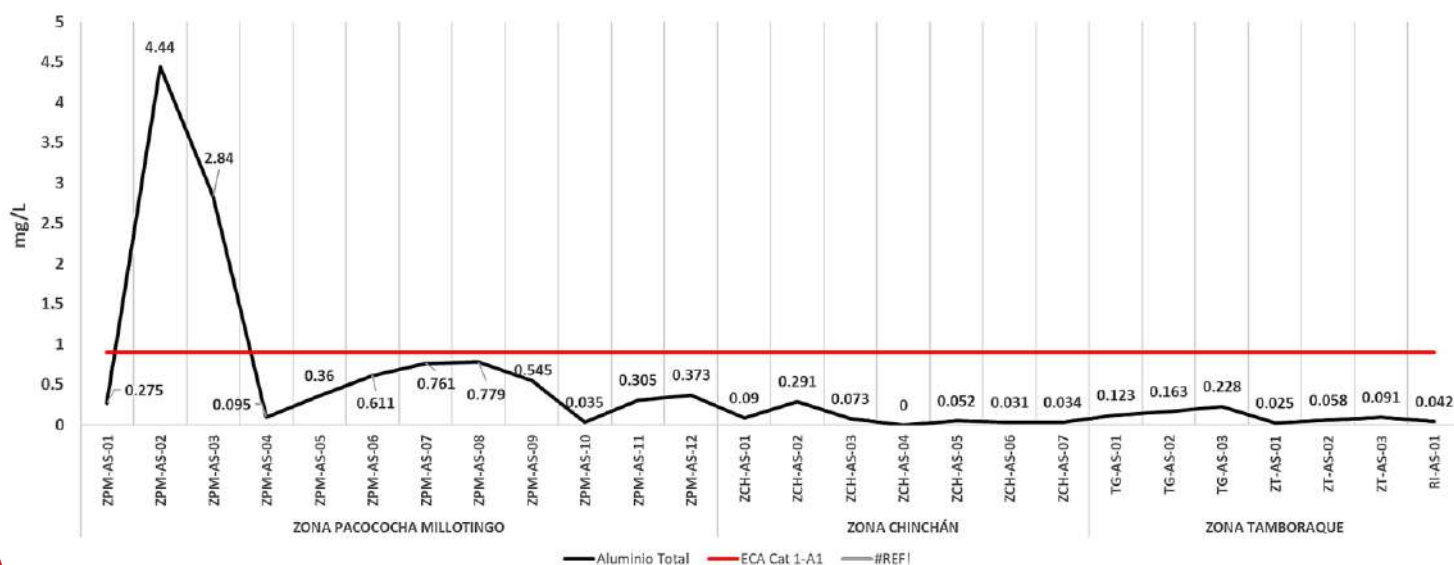
Gráfico N° 02. Valores de aluminio en aguas superficiales para las tres zonas.
