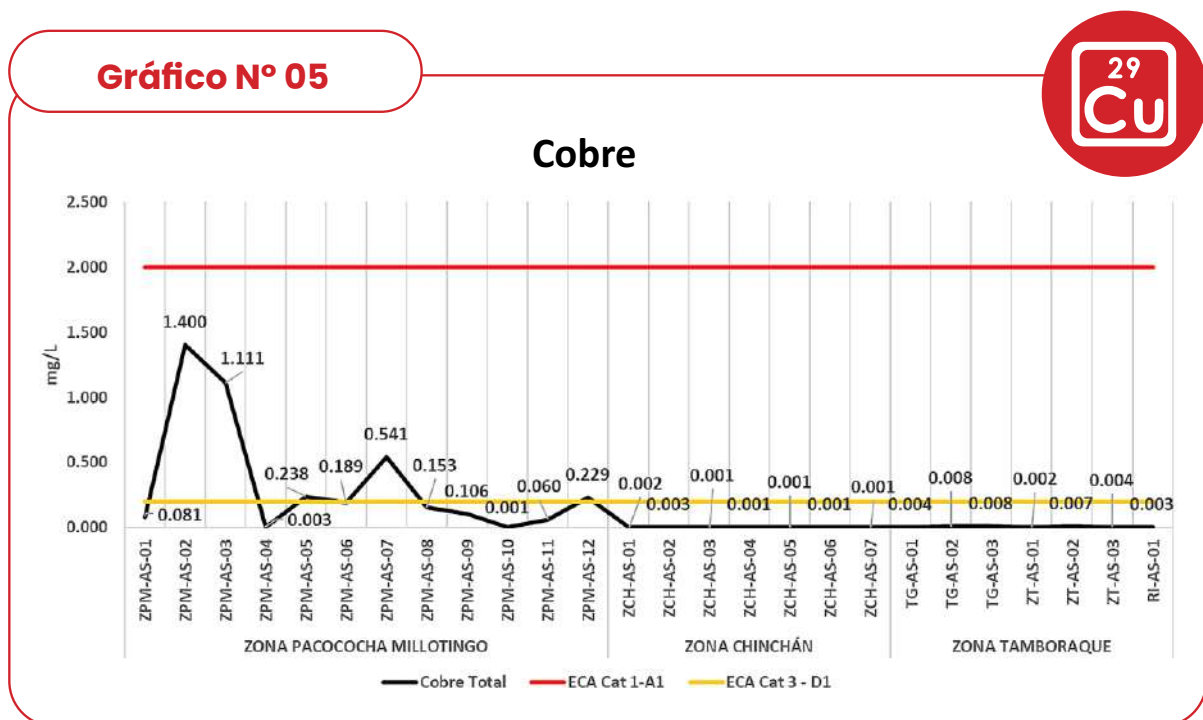
Gráfico N° 05. Valores de cobre en aguas superficiales para las tres zonas.
