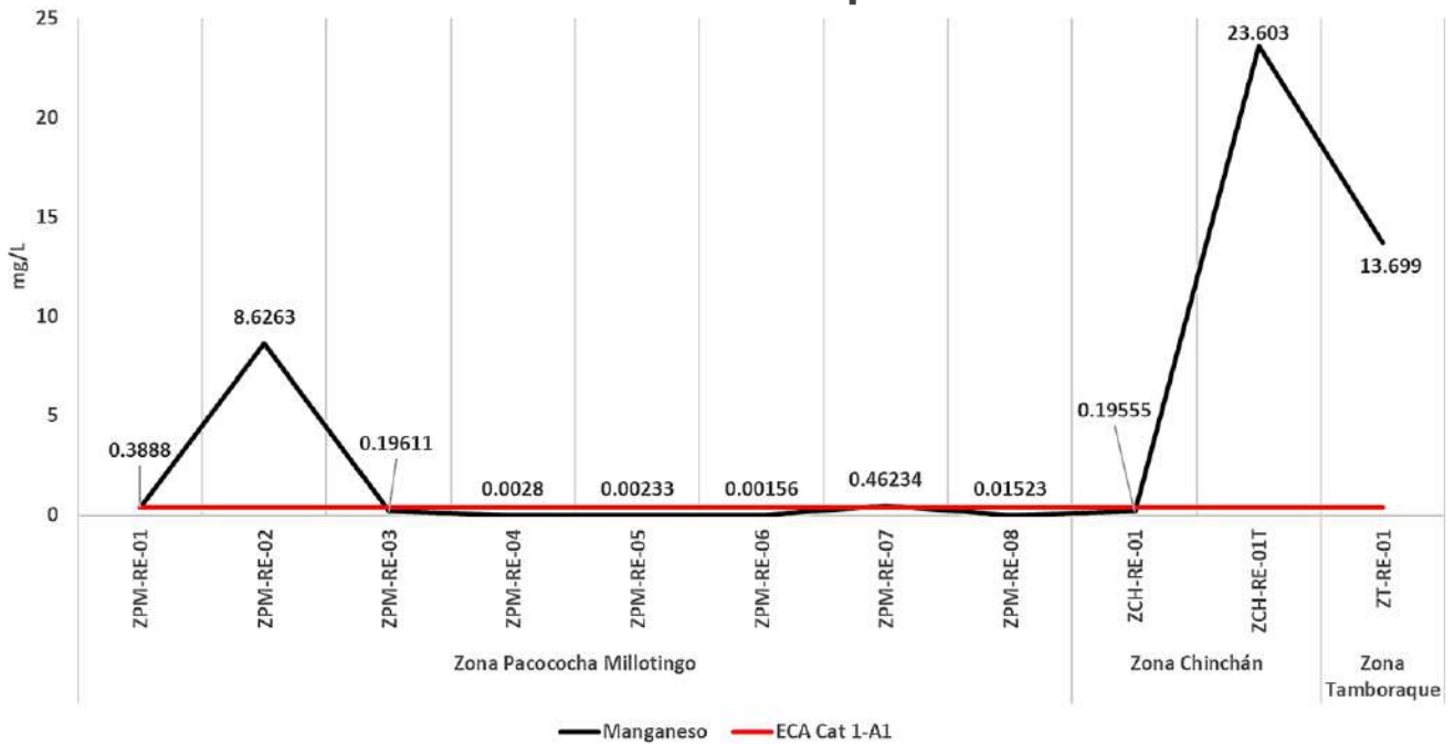
Gráfico N° 24. Valores de manganeso según Prueba de Lixiviados de Corto Plazo
