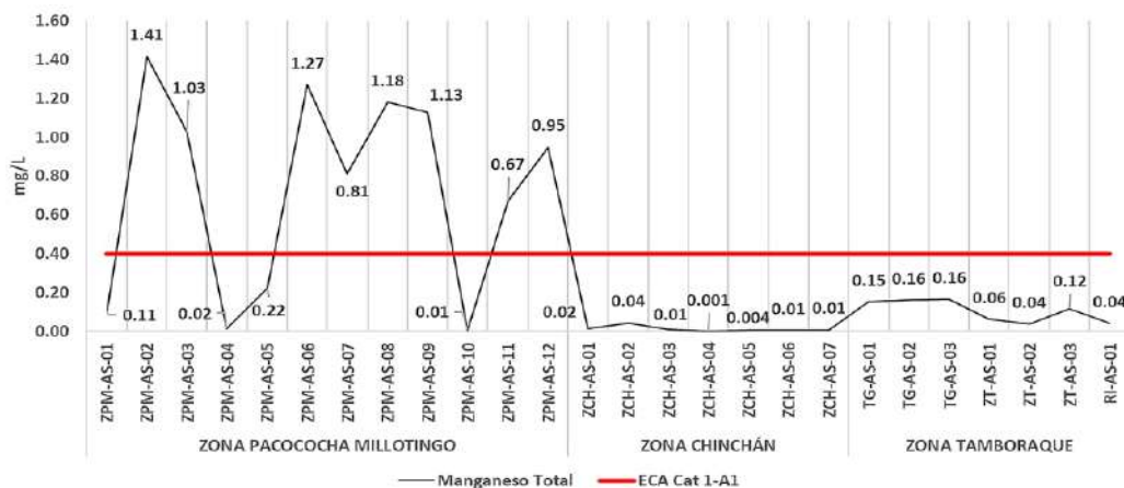
Gráfico N°07. Valores de manganeso en aguas superficiales para las tres zonas.
