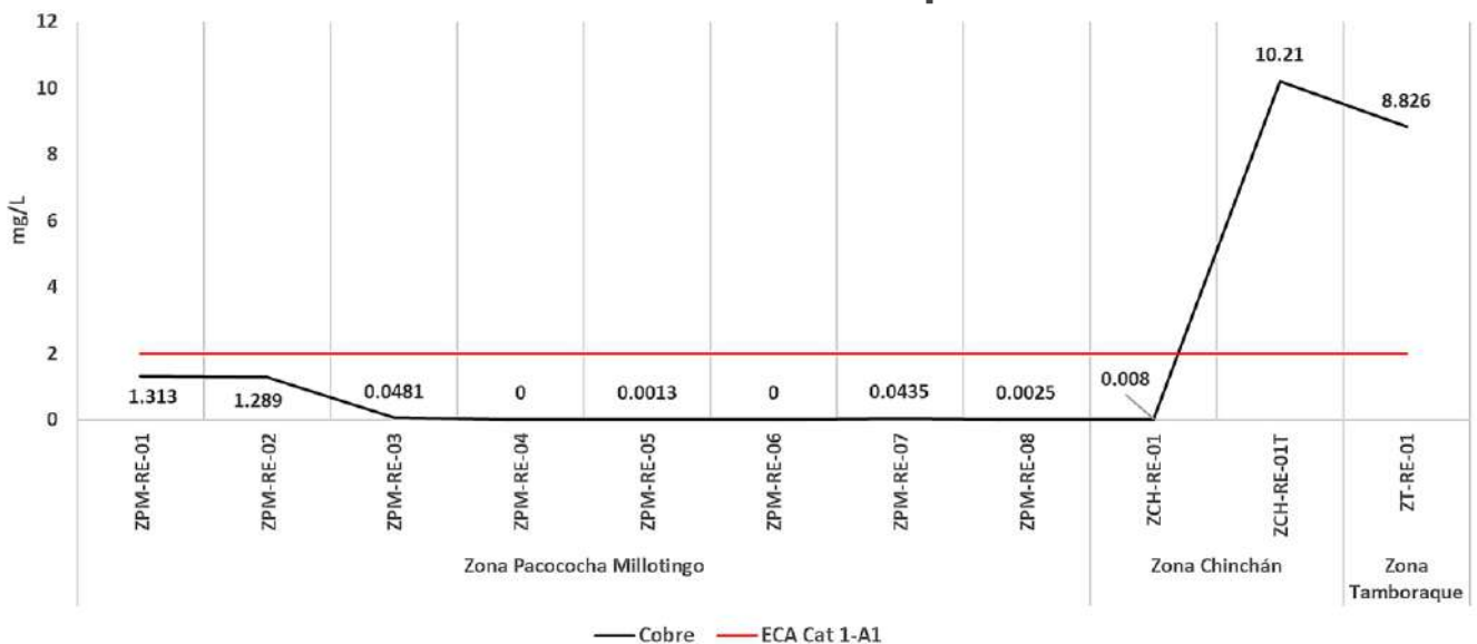
Gráfico N° 21. Valores de cobre según Prueba de Lixiviados de Corto Plazo.
