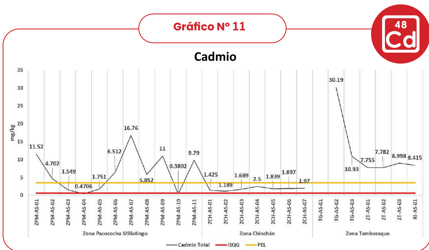
Gráfico N° 11. Valores de cadmio en sedimentos para las tres zonas.
