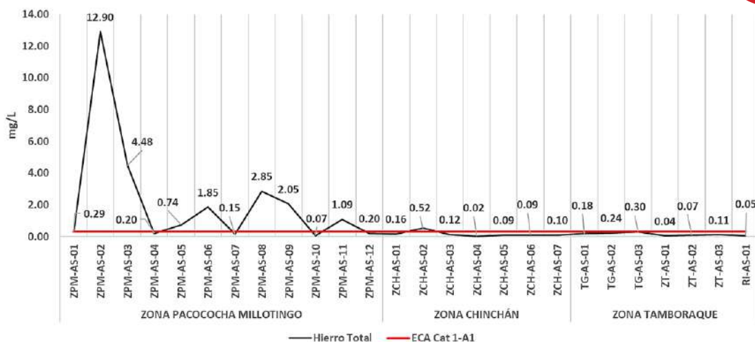
Gráfico N°06. Valores de hierro en aguas superficiales para las tres zonas.
