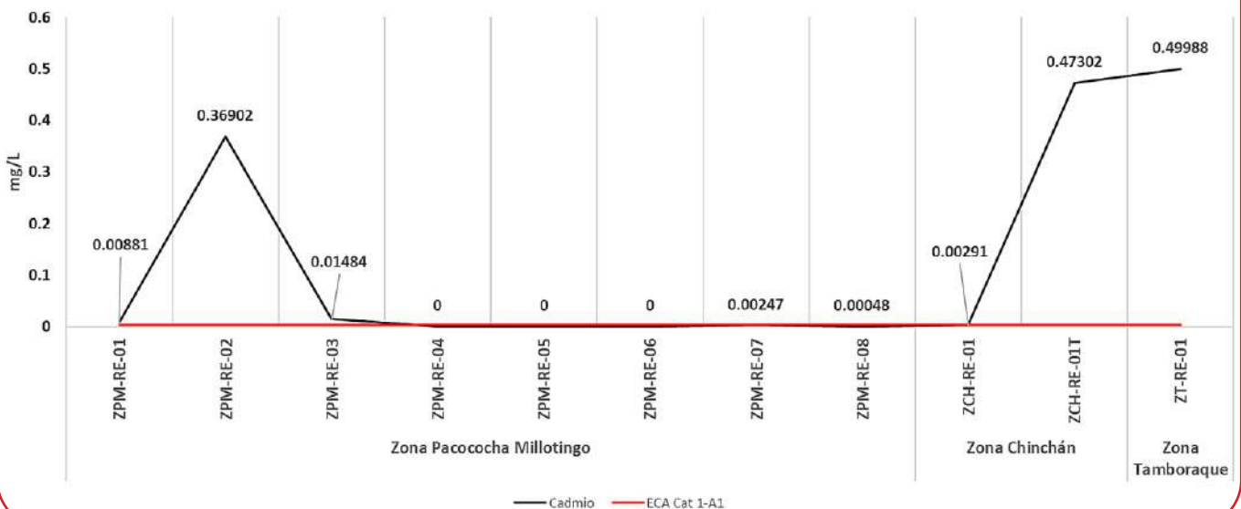
Gráfico N° 20. Valores de cadmio según Prueba de Lixiviados de Corto Plazo.
