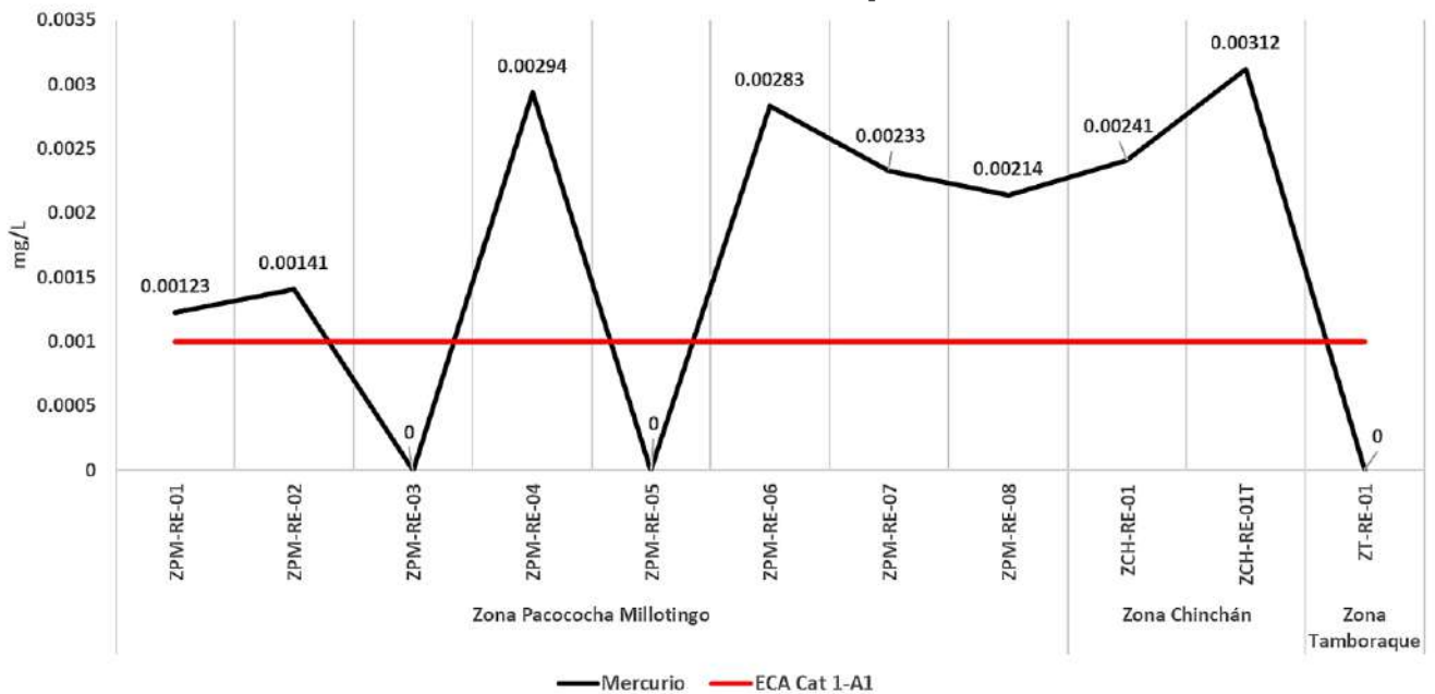
Gráfico N° 25. Valores de mercurio según Prueba de Lixiviados de Corto Plazo.
