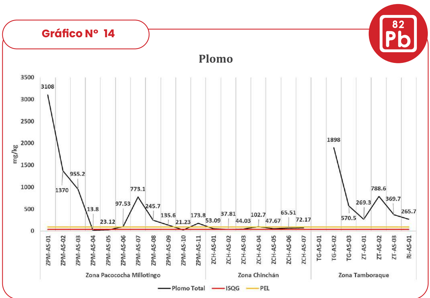
Gráfico N° 14. Valores de plomo en sedimentos para las tres zonas.
