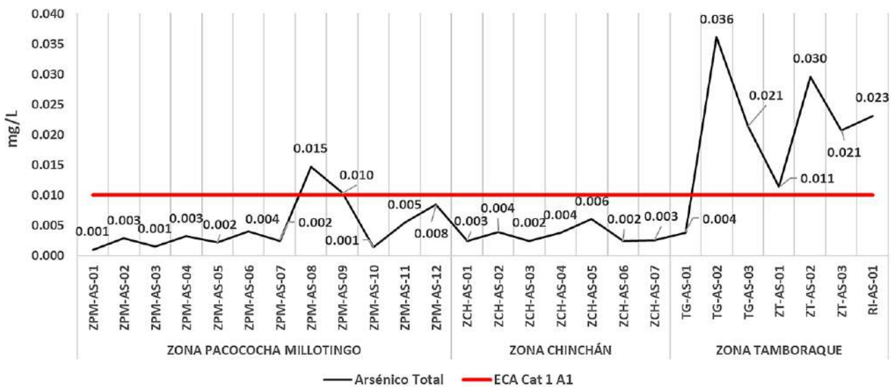
Gráfico N° 03. Valores de arsénico en aguas superficiales para las tres zonas.
