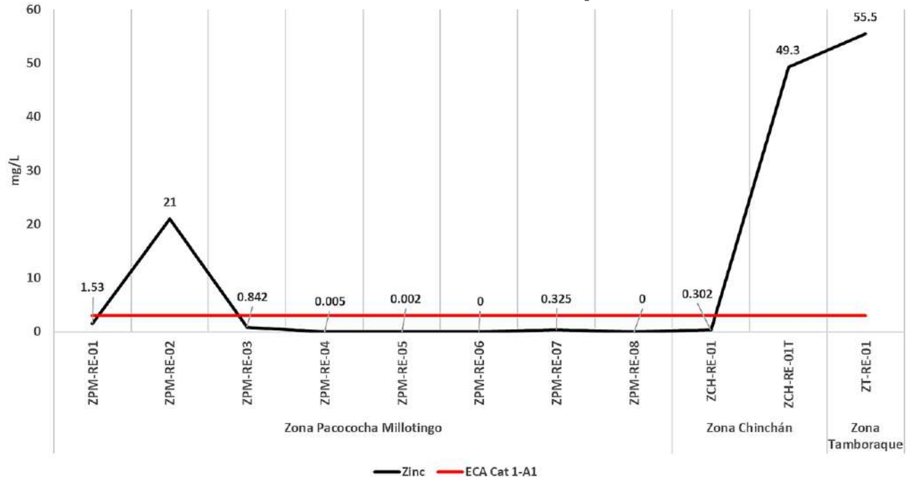
Gráfico N° 28. Valores de zinc según Prueba de Lixiviados de Corto Plazo
